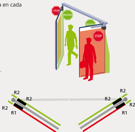
RELÉ 1: Señal de PARADA en el lado de apertura de la puerta.
