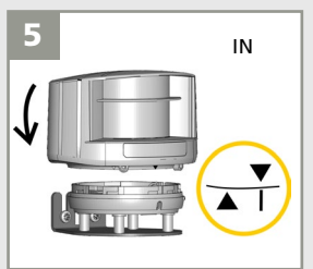
5 IN Posizionare l'involucro sulla staffa.
