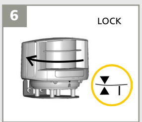
6 LOCK Ruotare il rilevatore finché i due triangoli non sono rivolti l'uno contro l'altro.
