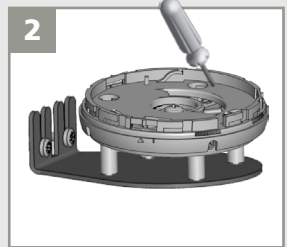
2 Posizionare la staffa e serrare a fondo le 4 viti per evitare vibrazioni.
