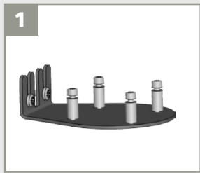
1 Utilizzare un montante o un accessorio di montaggio per fissare il rilevatore al palo (accessorio LBA, ad esempio).
